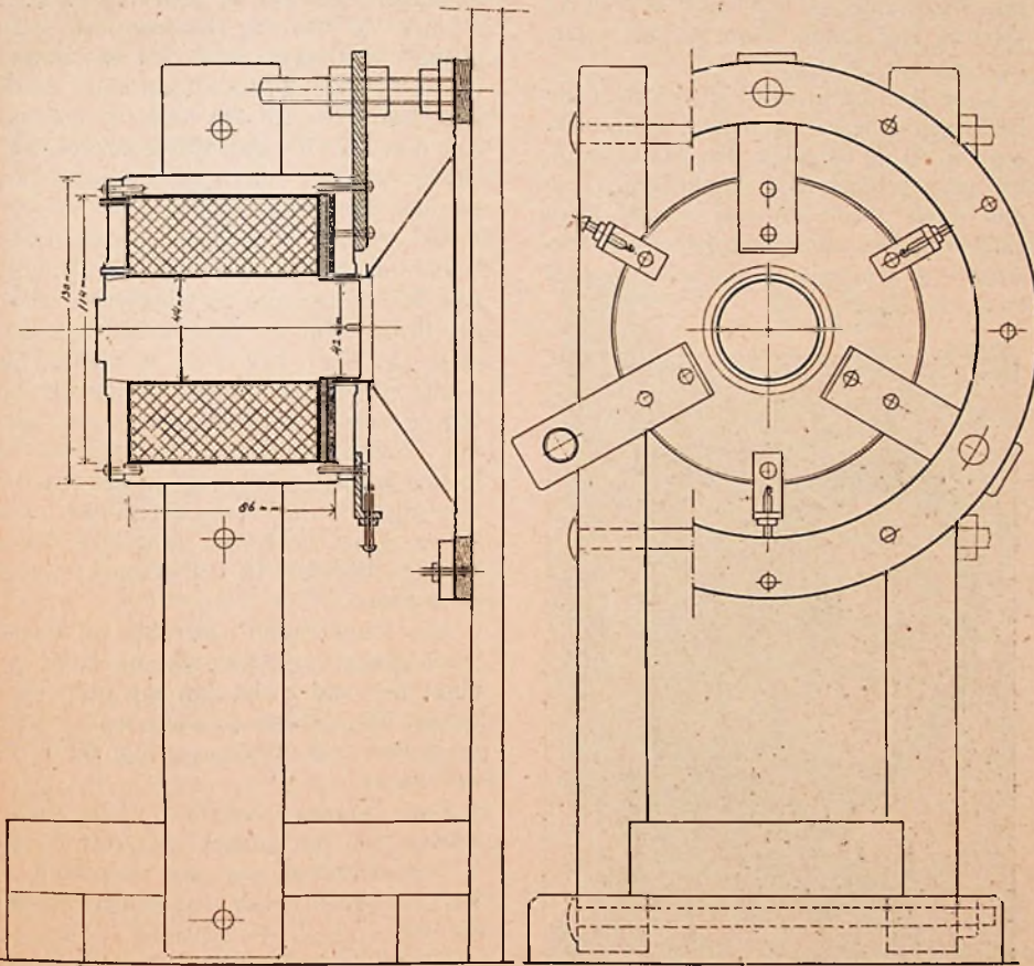
Fig. 1. Constructietekening.
